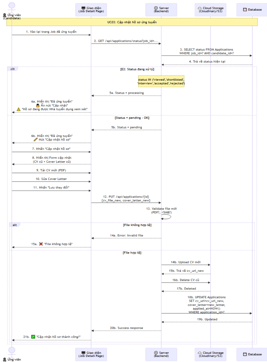
Hình ảnh thiết kế UC03:
